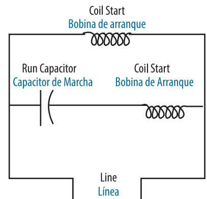
Reference installation diagram Diagrama de instalación de referencia
